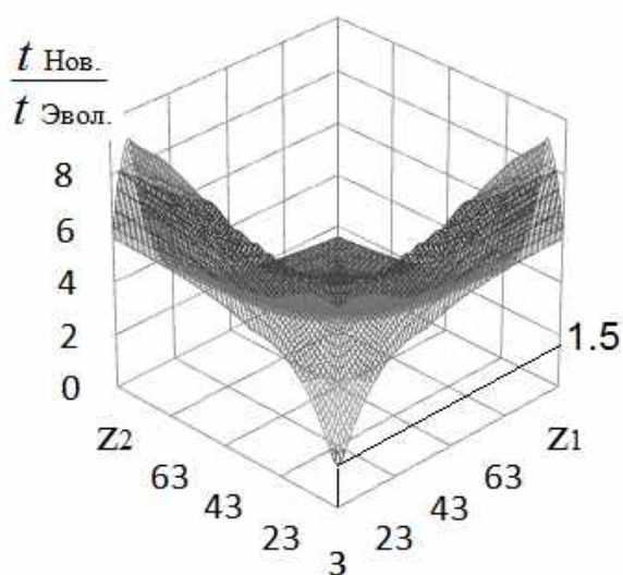
Рис. 22. Сравнение зацеплений ( \beta=20^\circ ; \sigma_{Hlim1}/S_{1H} = 500 МПа; \sigma_{Fim1}/S_{1F} = 290 МПа)
