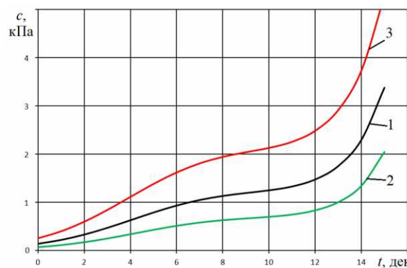
Рис. 5. Зависимость изменения связности снега от времени (декады)
