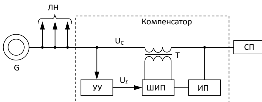
Рис. 1. Функциональная схема компенсатора нелинейных искажений напряжения
