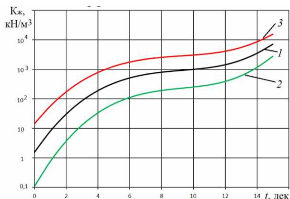
Рис. 4. Зависимость изменения коэффициента жесткости снега от времени (декады)
