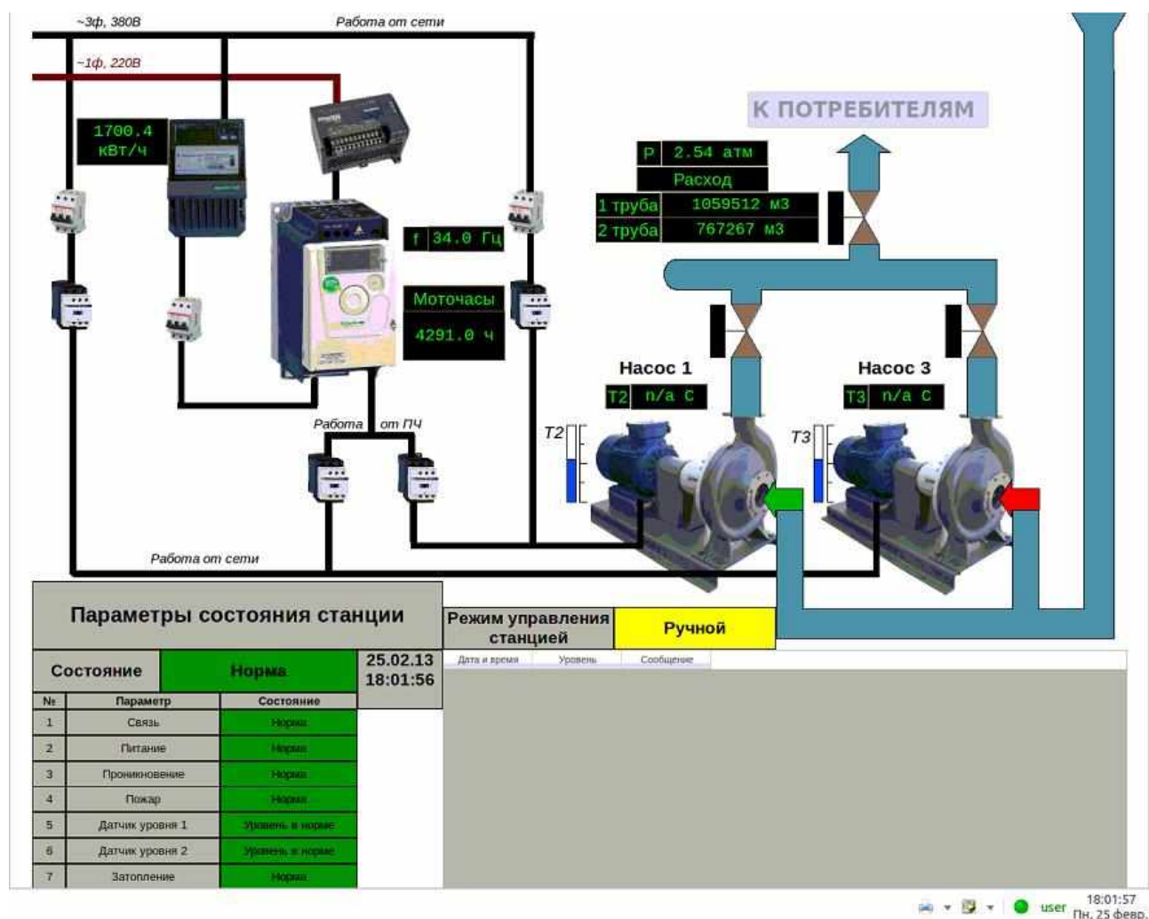
Рис. 3. Пользовательский интерфейс насосной станции г. Егорьевск Московской области
