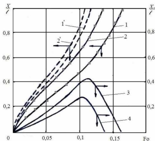
Рис. 2. Кривые продвижения изотерм солидуса и ликвидуса (пунктирные кривые) и развития ДЗ непрерывнолитого стального слитка сечением 330х360 при скорости вытягивания 0,5 м/мин:
