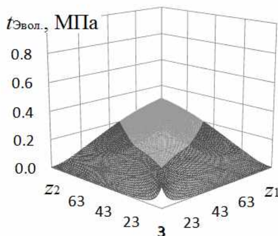
Рис. 21. Лимитирующая нагрузочная способность эвольвентного зацепления ( \beta=20^\circ ; \sigma_{Hlim1}/S_{1H} = 500 МПа; \sigma_{Fim1}/S_{1F} = 290 МПа)
