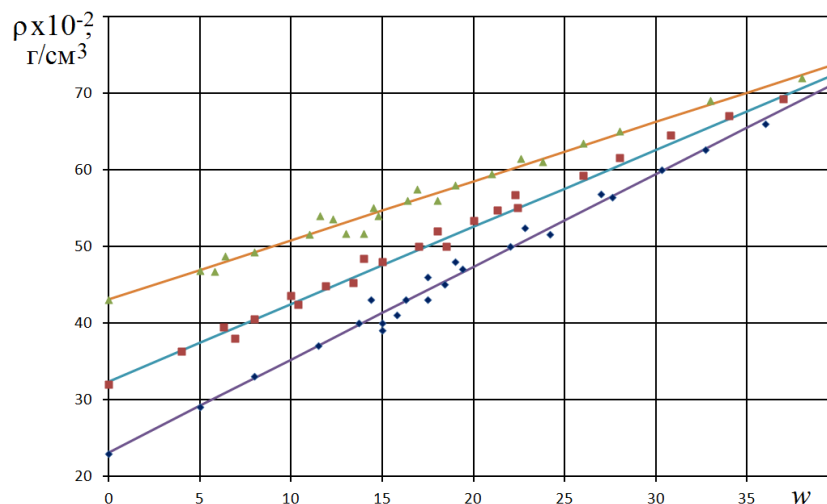
Рис. 7. Зависимость плотности от влажности: точками показаны экспериментальные данные, линиями – теоретические
