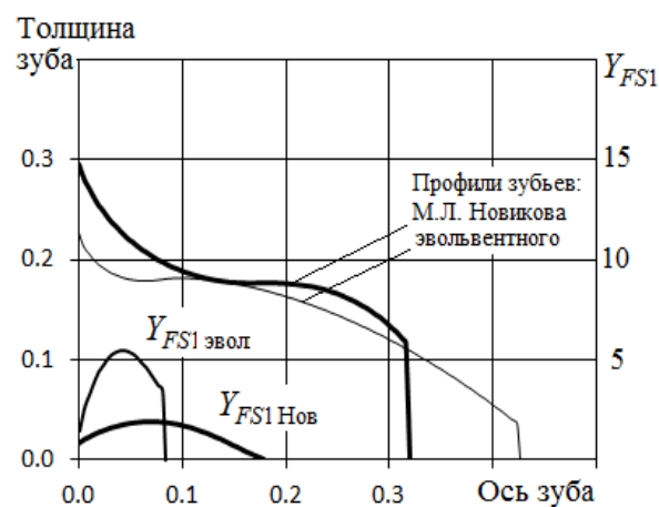
Рис. 23. Профили зубьев и эпюры коэффициентов формы зубьев шестерни для z_1=10 , z_2=36
