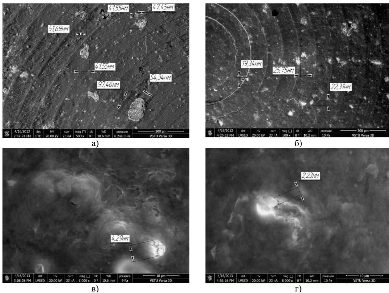
Рис. 3. Микрофотографии 7 мас.% водно-глинистой суспензии без добавления УЦР (а, в), с добавлением 1 мас.% УЦР (б, г); а, б – \times 500 ; в, г – \times 8000
