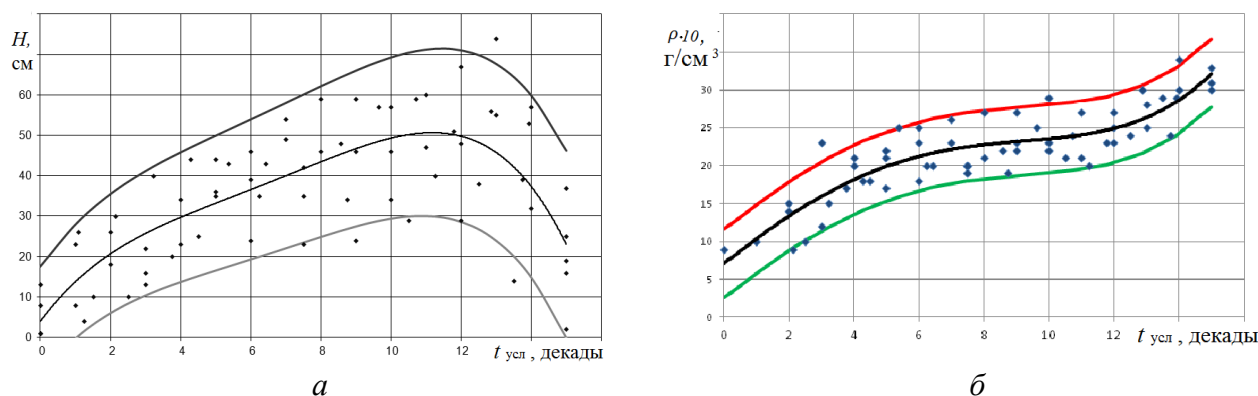
Рис. 3. Пример изменения характеристик снежного покрова в зависимости от условной продолжительности зимнего периода, полученные по результатам многолетних наблюдений: а – глубина; б – плотность
