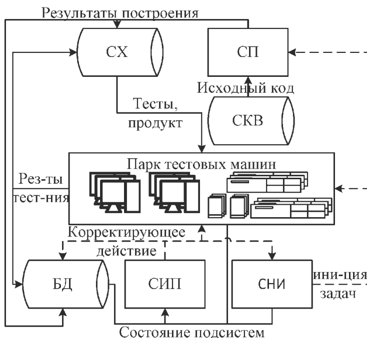
Рис. 1. Архитектура системы
