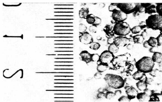
Рис. 2. Зернистая структура снежного покрова
