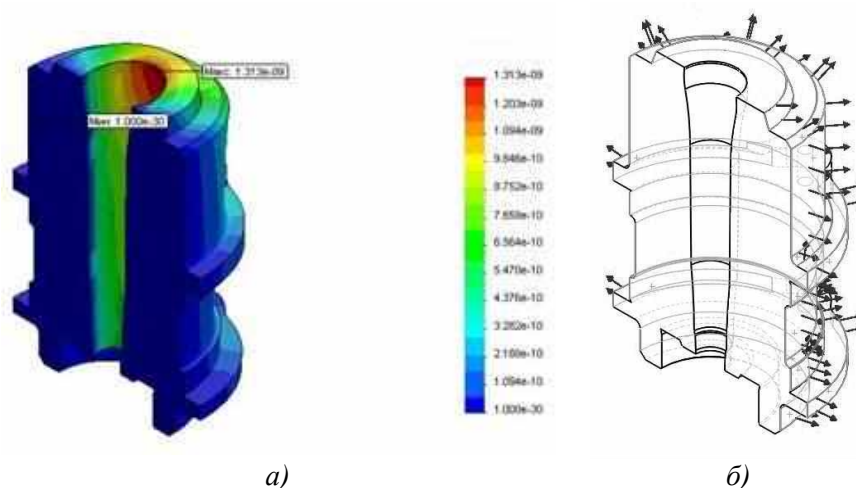
Рис. 3. Схема напряженного состояния детали стеклоформы:
