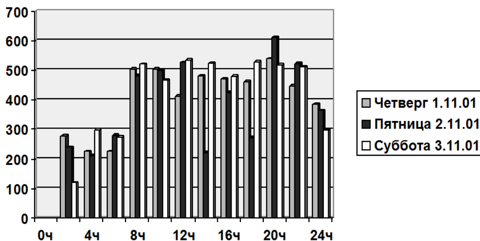
Рис. 1. График водопотребления
