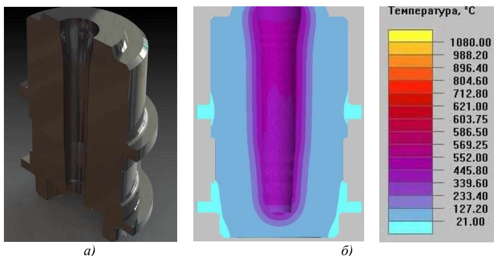
Рис.2. Стеклоформирующая оснастка:
