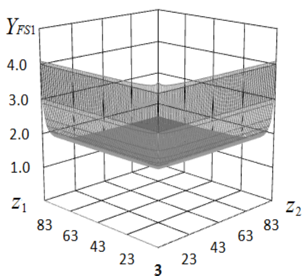
Рис. 17. Коэффициентов формы зуба шестерни
