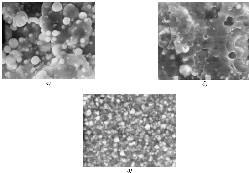
Рис. 5. Электронные микрофотографии поверхностной структуры покрытий: а, б - TiN (x5000); в - TiC+Ti(C-N)+Al 2 O 3 (x5000)
