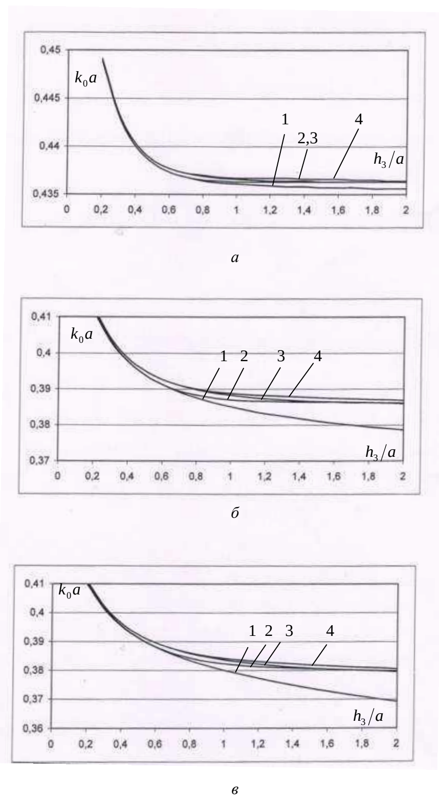
Рис. 2. Графики зависимости резонансного волнового числа от положения верхней крышки экрана при различных значениях его диаметра: a - b/a = 1,2 ; б - b/a = 2,0 ; в - b/a = 5,0
