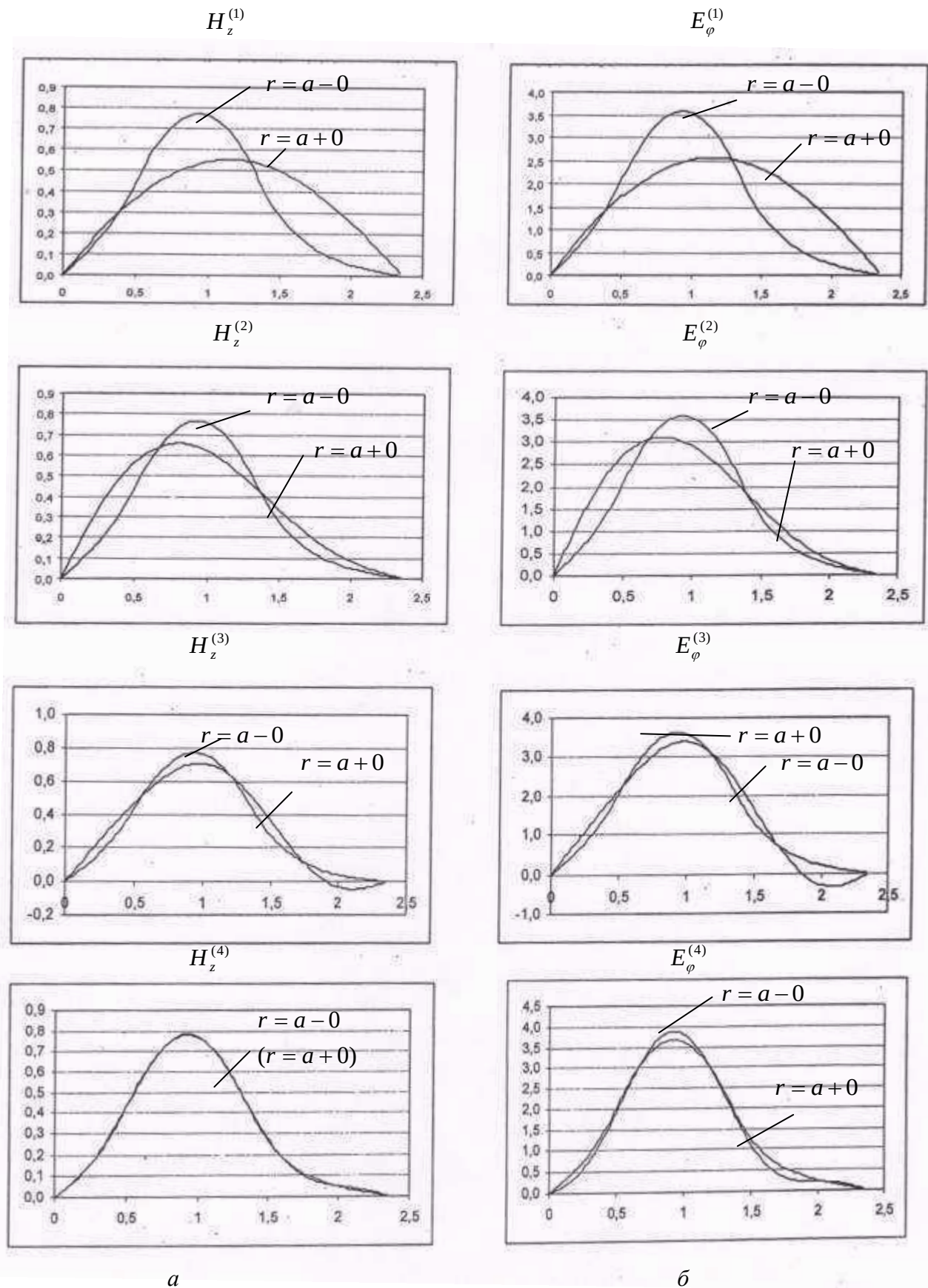
Рис. 4. Графики зависимости от величины z/a компонент электромагнитного поля в резонаторе на цилиндрической границе r = a при большом размере экрана ( b/a = 5,0 )
