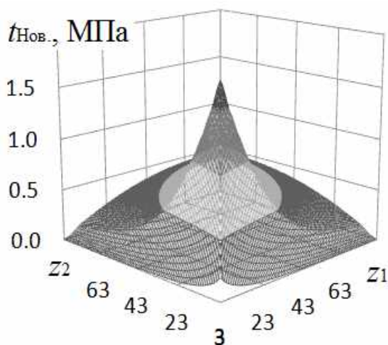
Рис. 20. Лимитирующая нагрузочная способность зацепления М.Л. Новикова ( \beta=20^\circ ; \sigma_{Hlim1}/S_{1H} = 500 МПа; \sigma_{Fim1}/S_{1F} = 290 МПа)
