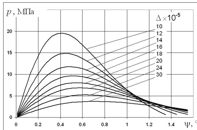
Рис. 11. Давление в гидродинамическом слое ( \eta = 0.5 \text{ Па} \cdot \text{с} , \omega = 100 \text{ с}^{-1} , k = 0,25 )
