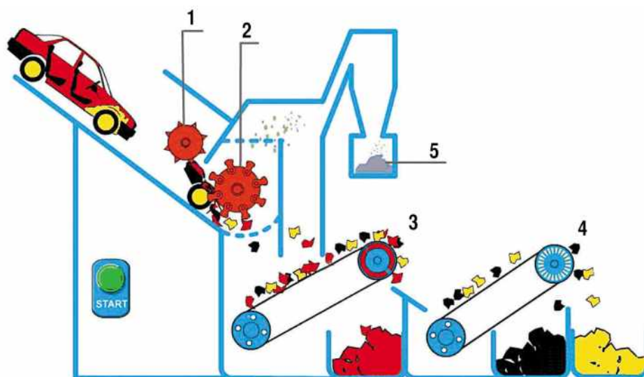
Рис. 2. Схематичное изображение шредерной установки:
