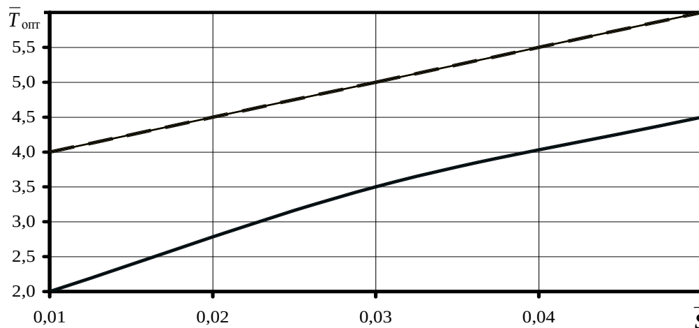
Рис. 2. Зависимость оптимального относительного натяжения от относительного статического смещения ППБУ при глубине моря 75 м: ————— V_0 = 0 , — — — — V_0 = 1 м/с
