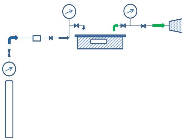
Рис. 2. Схема проточной системы для анализа состава генераторного газа методом Фурье ИК-спектроскопии
