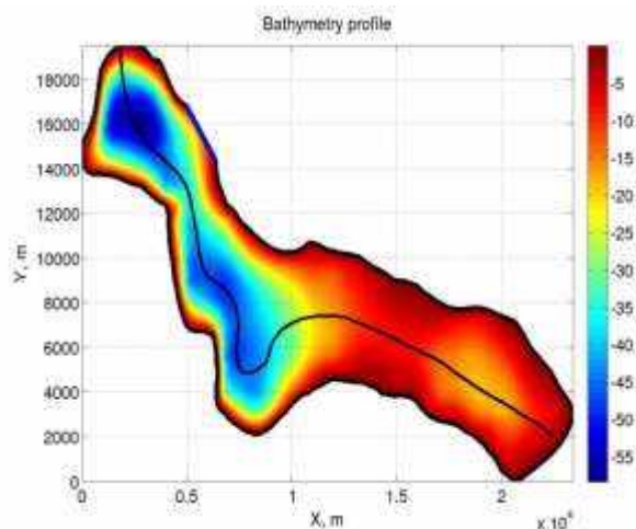
Рис. 11. Батиметрия озера Тунайча: черной кривой обозначен профиль, под которым проводился замер гидрологических параметров в численной модели
