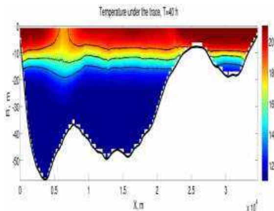
Рис. 10. Распределение профиля температуры
