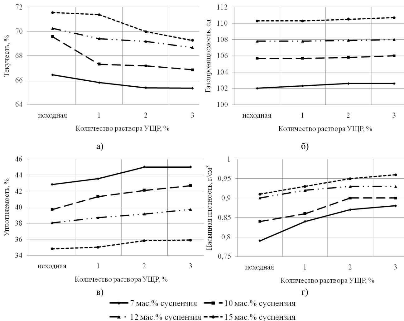
Рис. 5. Влияние УЦР на свойства формовочных смесей с добавлением водно-глинистых суспензий различной концентрации а – текущность (по Орлову Г.М.); б – газопроницаемость; в – уплотняемость; г – насыпная плотность
